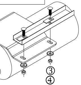
Isolateur en caoutchouc non illustré
