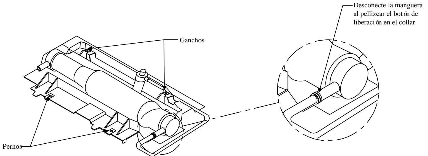
Figura 2 Recipiente de carbono
