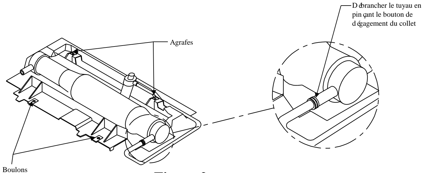
Figure 2 Absorbeur de vapeurs d'essence
