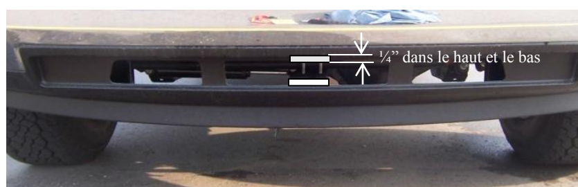
Découper le carénage comme illustré FIG.2
